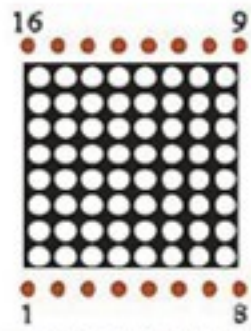
数码管显示及引脚位置图
